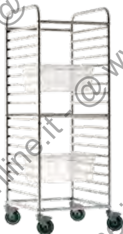
111236 - CARRELLO PORTATEGLIE INOX CM 73X62X171 PER 18 TEGLIE 2/1 H 65 OPPURE 36 TEGLIE 1/1 H 65 PORTATA KG 300
